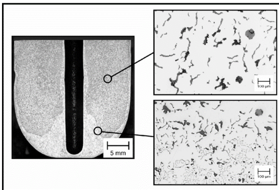
Рис. 7. Моделирование влияния исчезновения магния в чугуна
