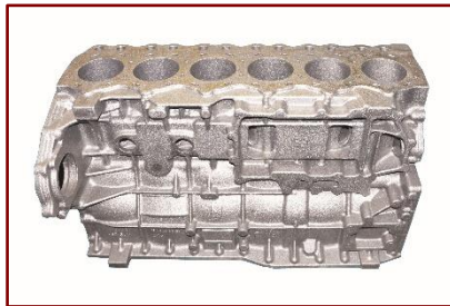
9.0 리터 SinterCast-CGI 엔진블록
